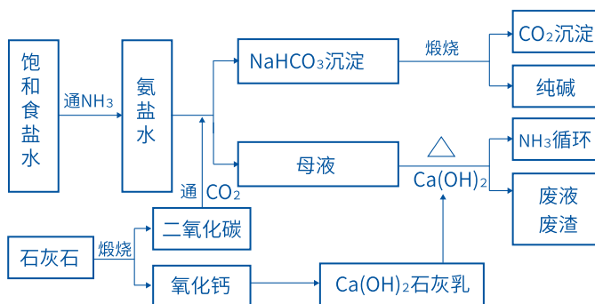
图 1-3 氨碱法纯碱生产流程图
